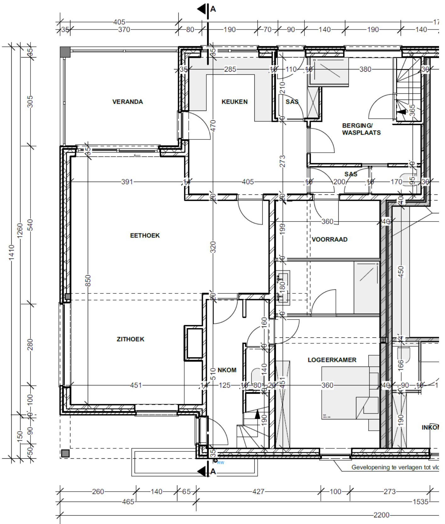
GRONDPLAN
