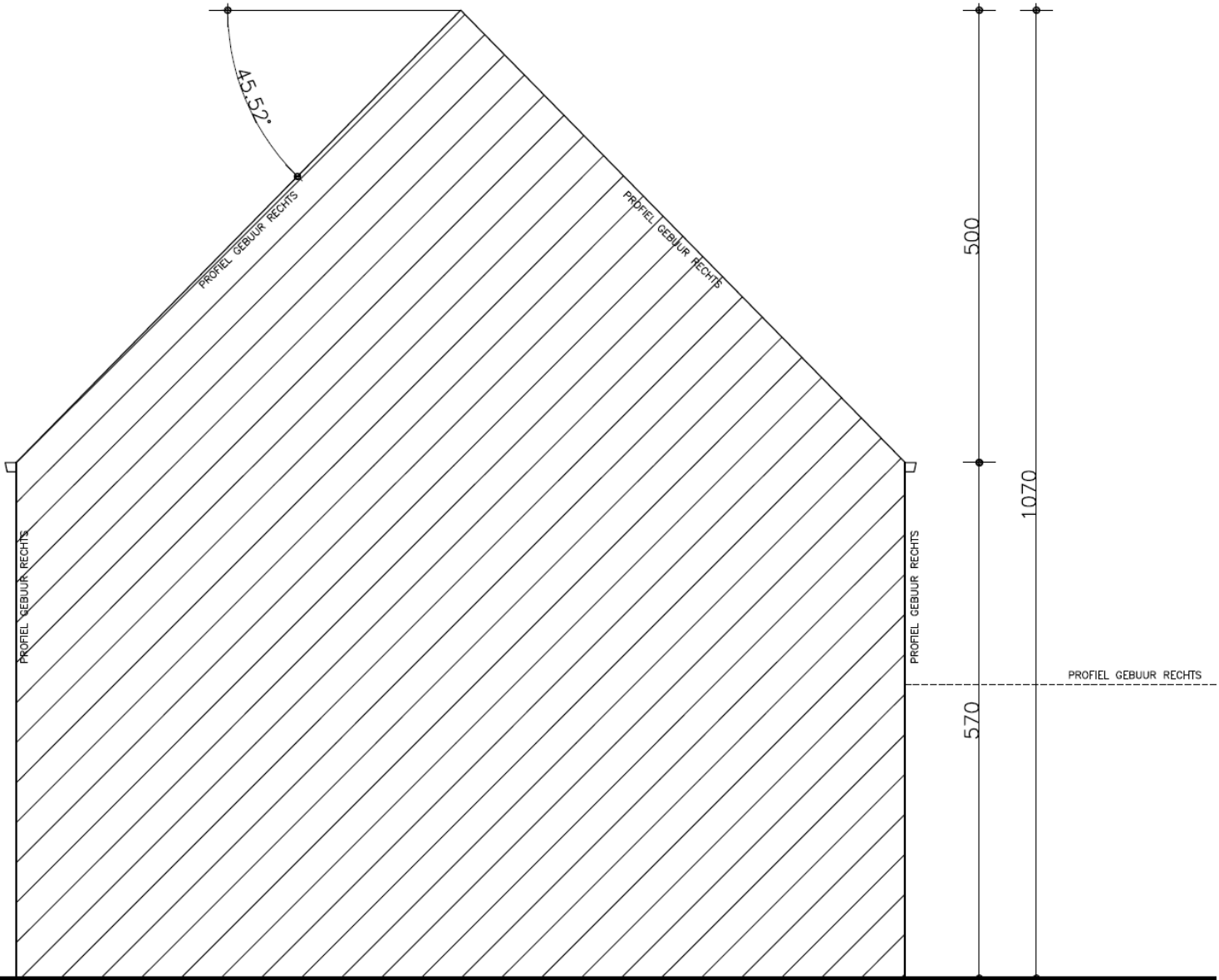
N ZIJGEVEL RECHTS sch. 1/50
