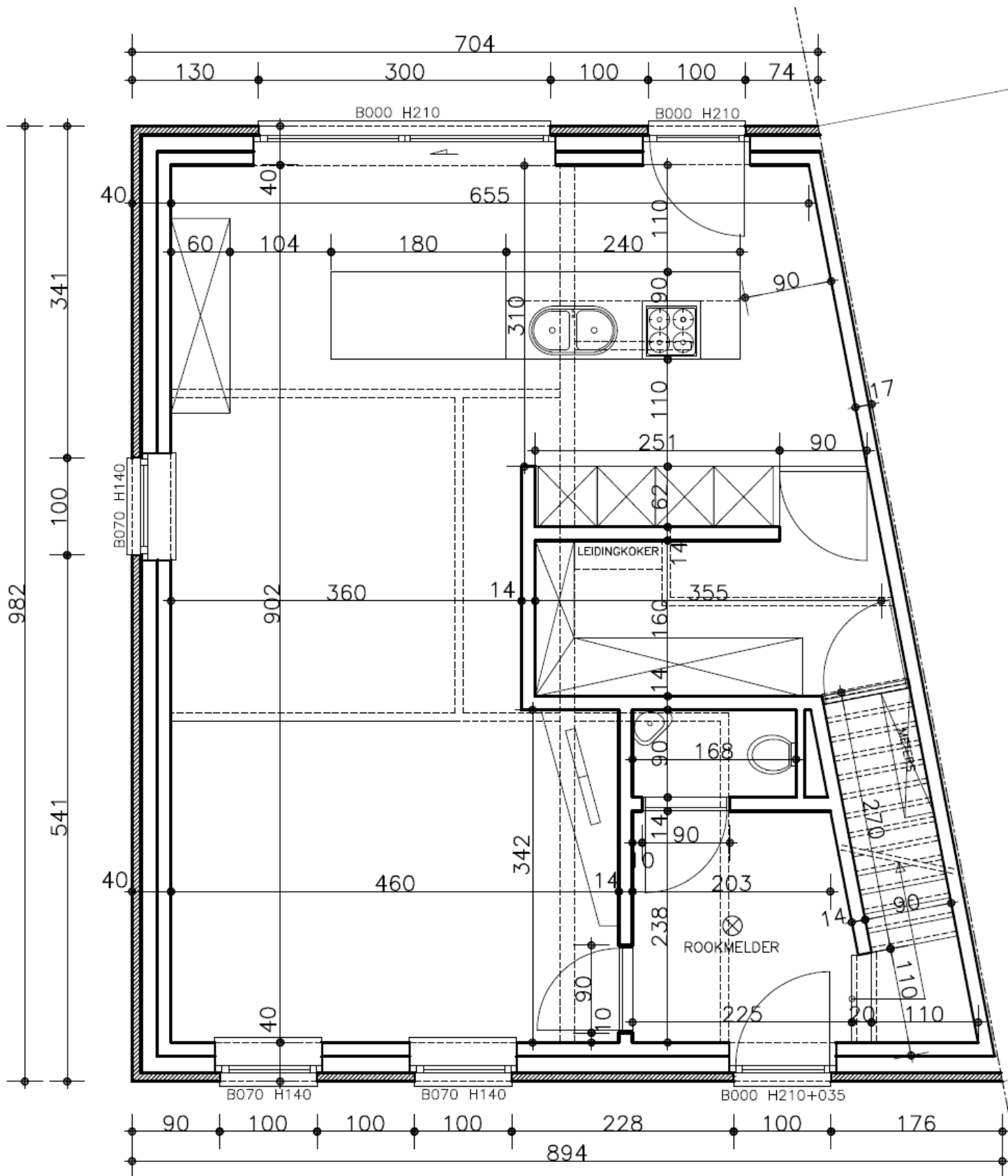
N GRONDPLAN sch. 1/50
