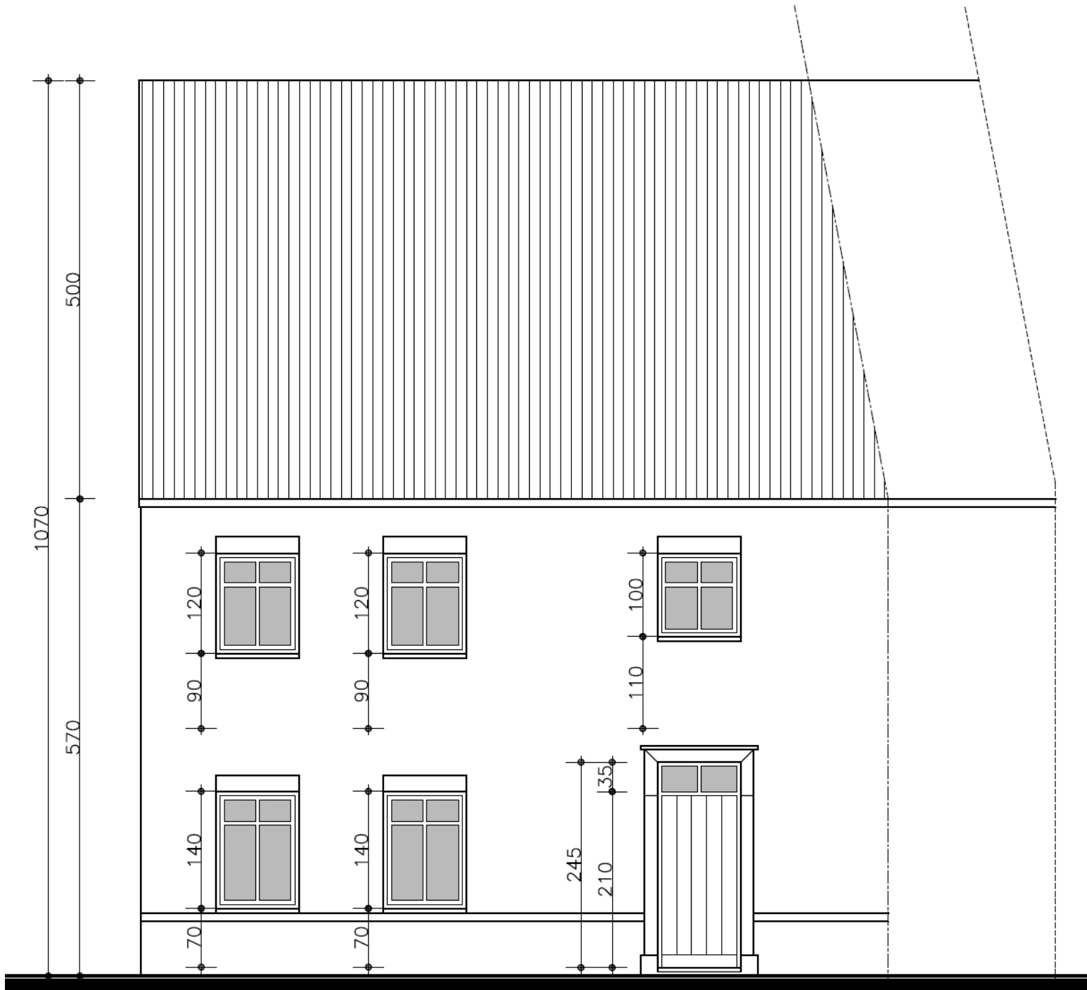
N VOORGEVEL sch. 1/50
