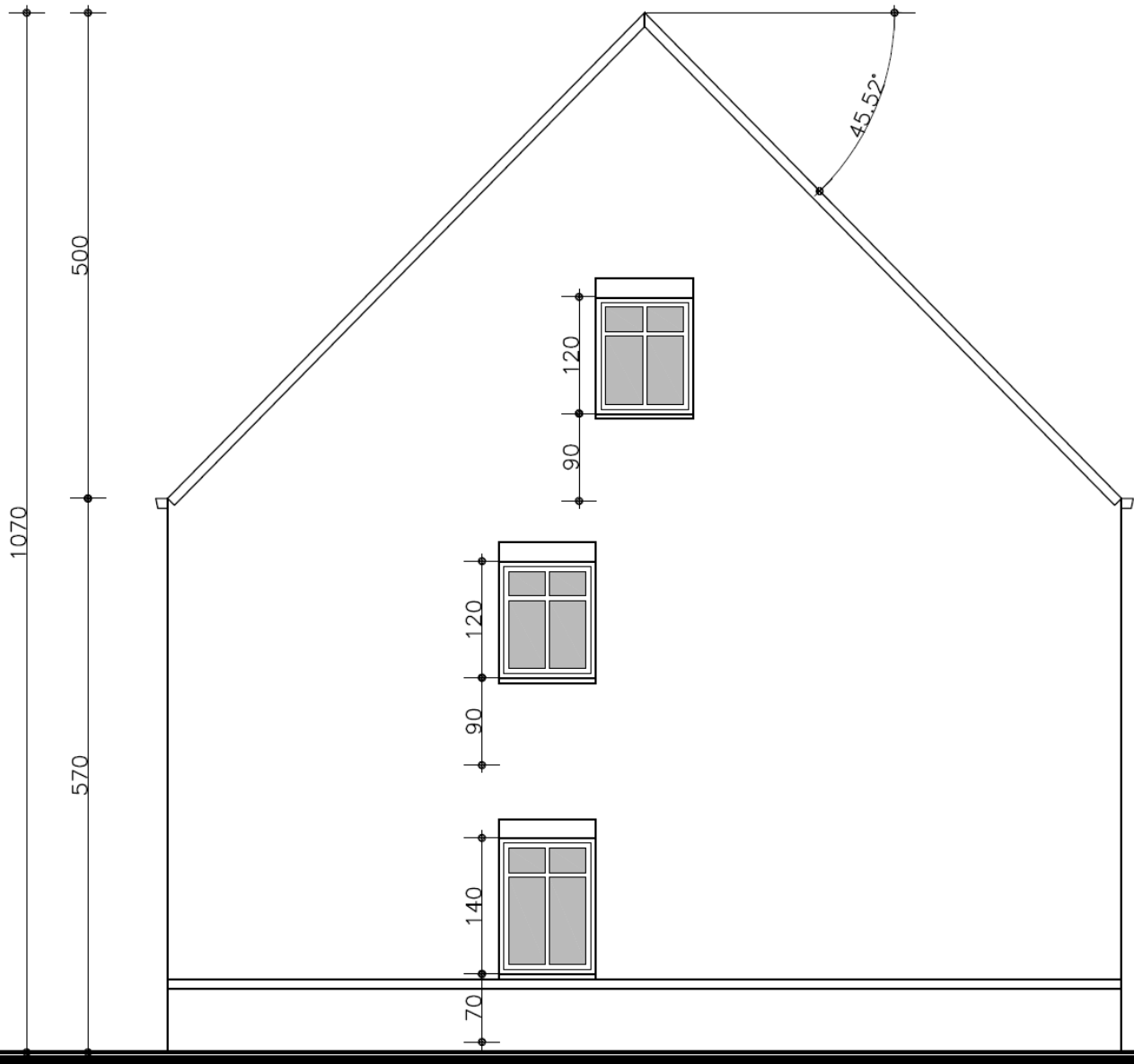
N ZIJGEVEL LINKS sch. 1/50
