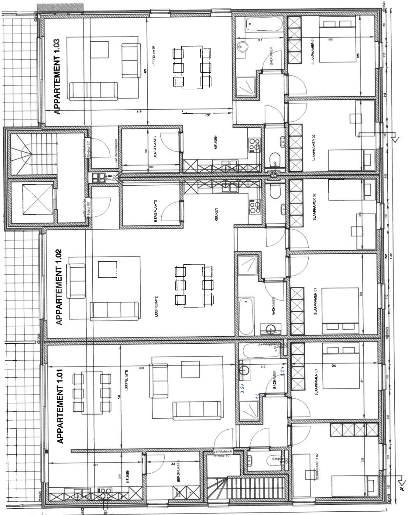
plan verdieninn + 1
