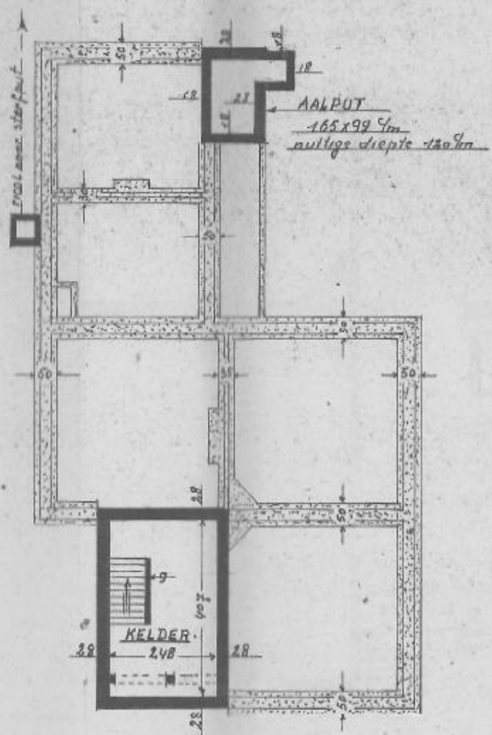
GRONDPLAN.
