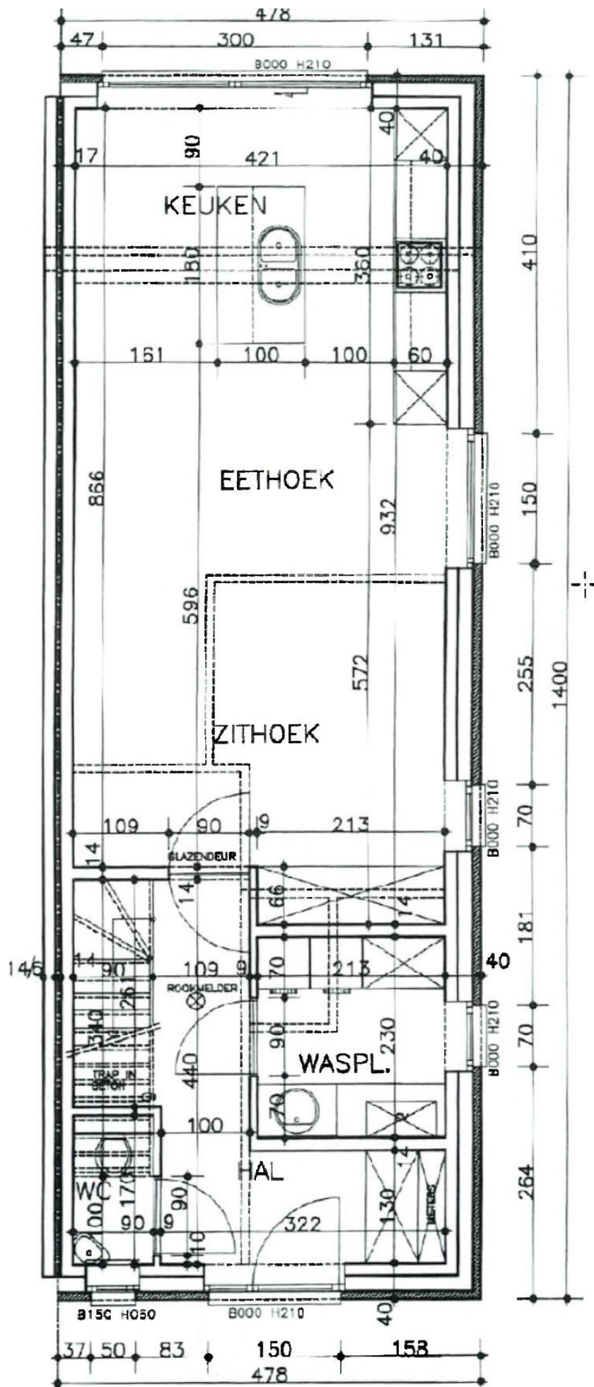
N GRONDPLAN sch. 1/50
